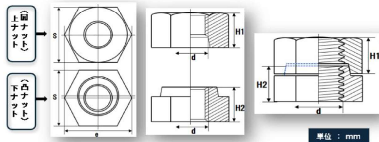
フジダブルロックナット®寸法表(ユニファイ)HEX(FIN)
